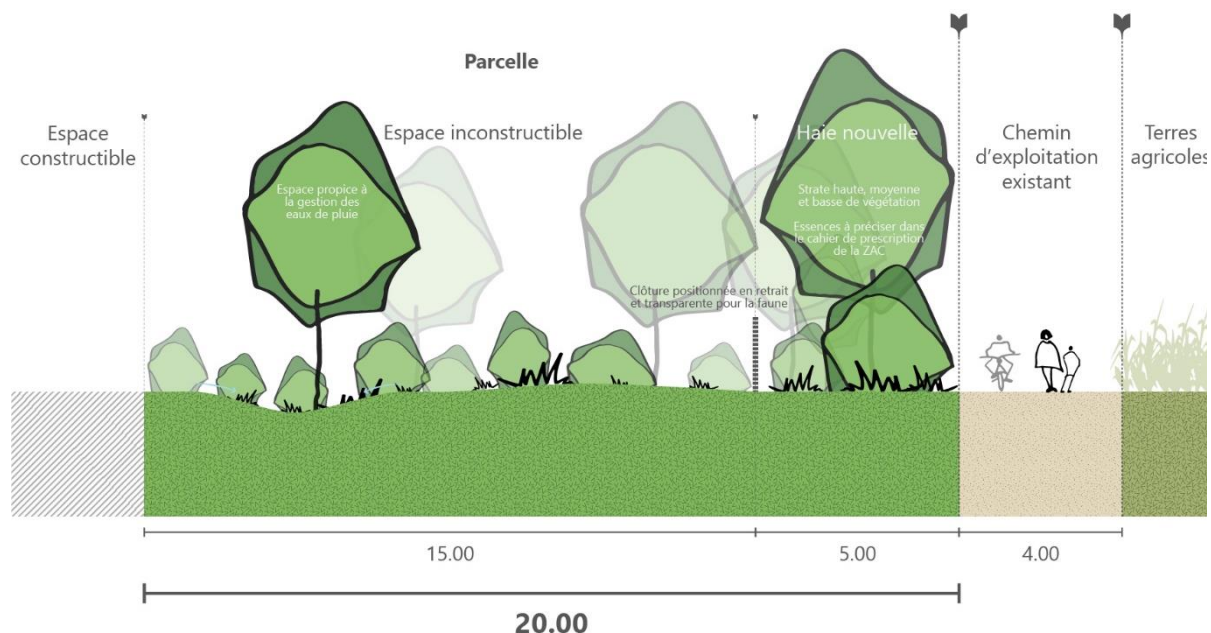
A - Localisation, principe d'aménagement des haies périphériques et profil en travers
