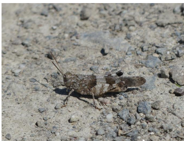
Conocéphale gracieux et Œdipode turquoise dans les aires d'études (BEE Ing, 10 août 2021)
