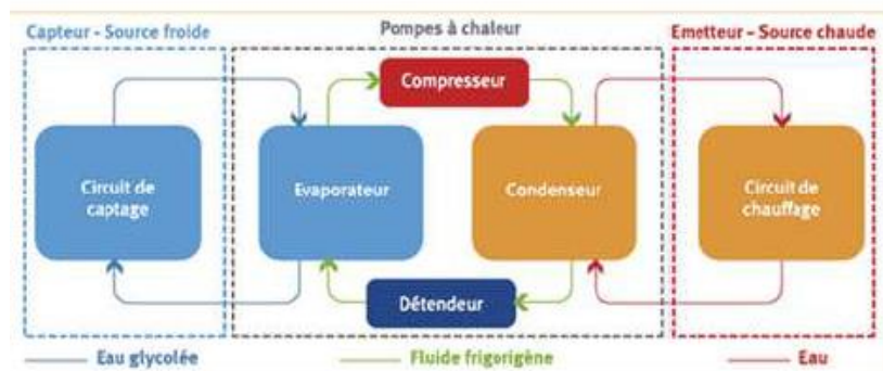
Pompe à chaleur eau/eau
