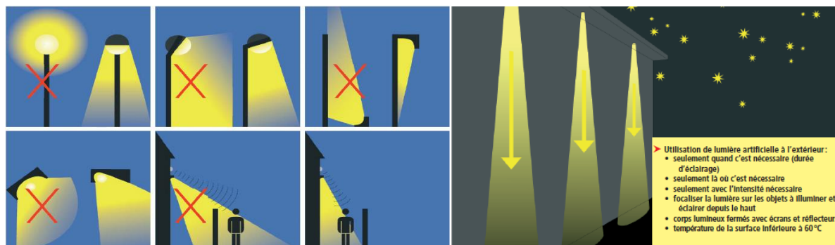
Figure 99 : Illustrations des techniques d'éclairage appropriées
