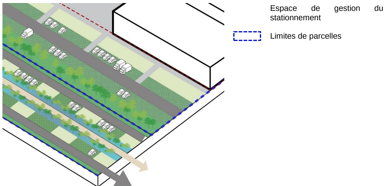
Figure 79 : traitement proposé pour le stationnement central public et le stationnement privé sur les parcelles
