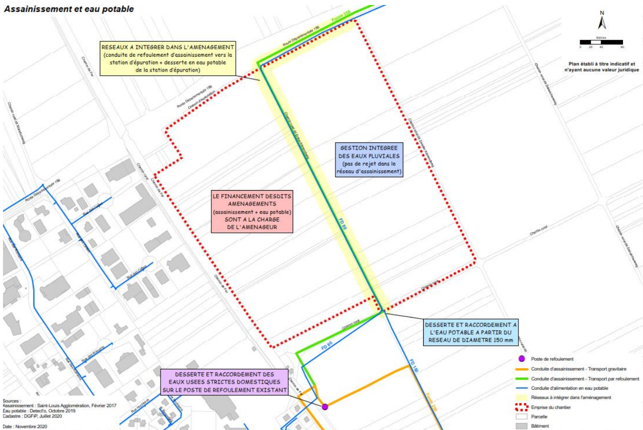
Figure 31 : Organisation actuelle des réseaux sur l'emprise du site et contraintes de desserte en réseaux – Source : Saint-Louis Agglomération
