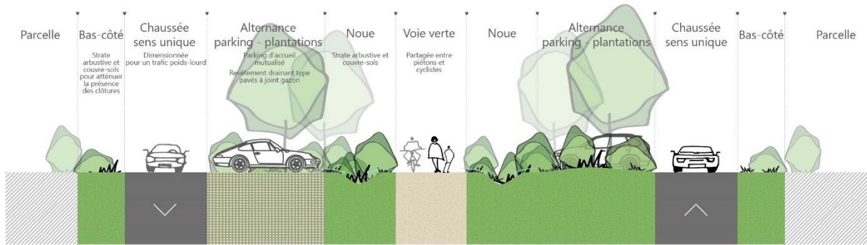
Figure 22 : coupe de la voie centrale pour la desserte de la zone d'environ 30 mètres de large
